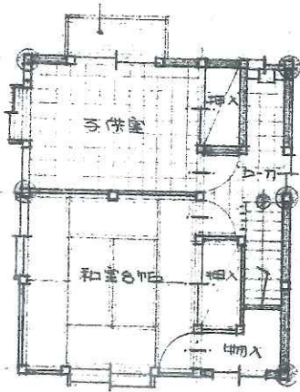
2階平面図 1/50
