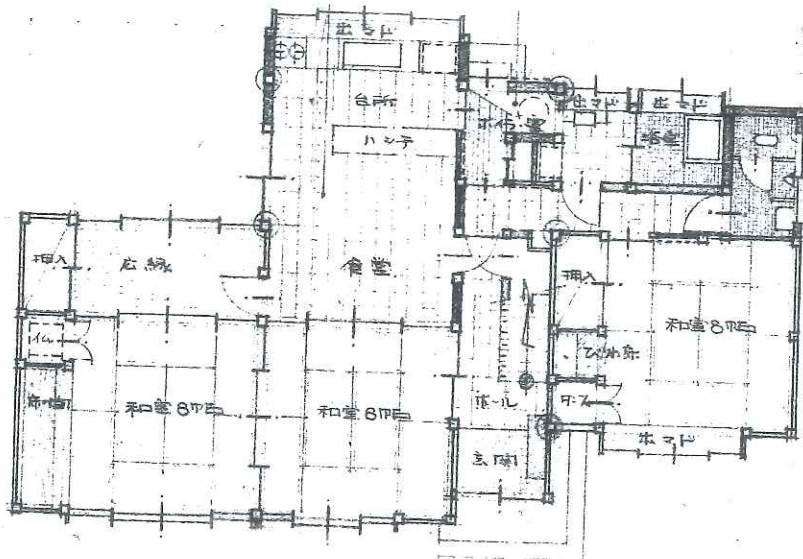
1階平面図 1/50
