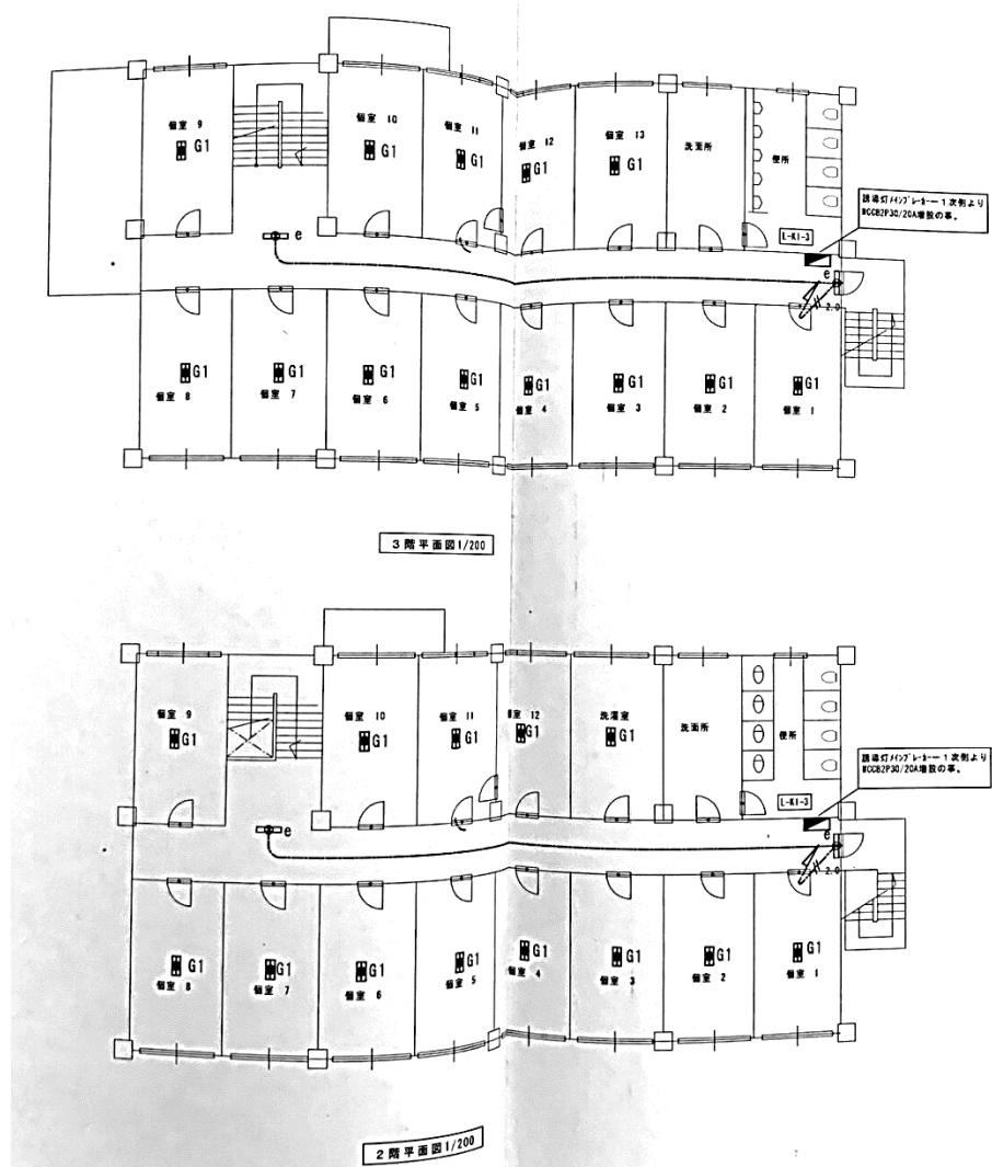
図面6 宿泊棟 2階・3階平面図
