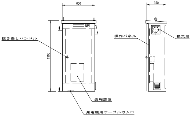
操作パネル図 (S=1/10)
