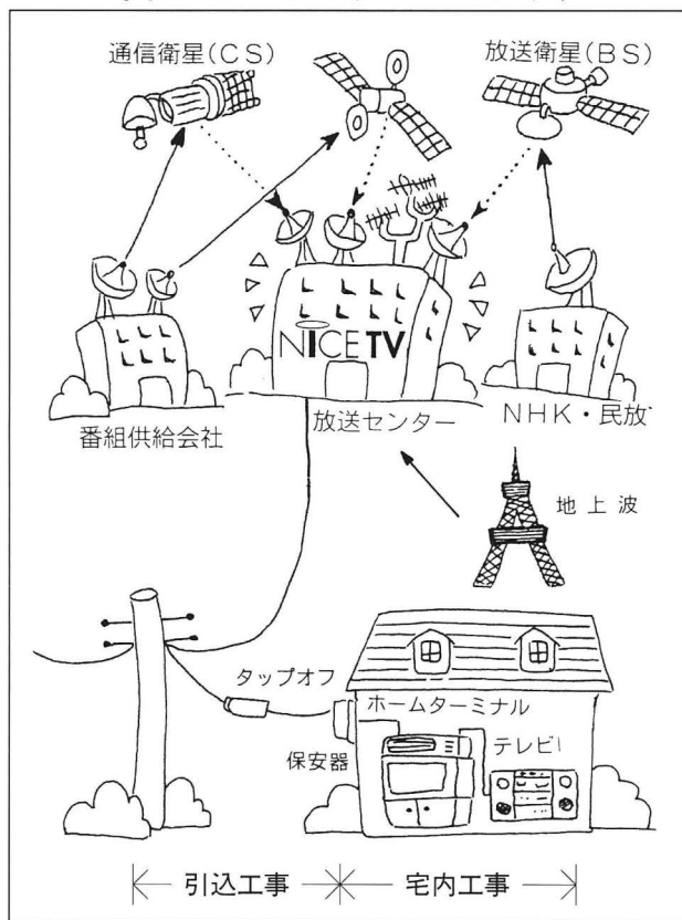
図1 ケーブルテレビのしくみ
