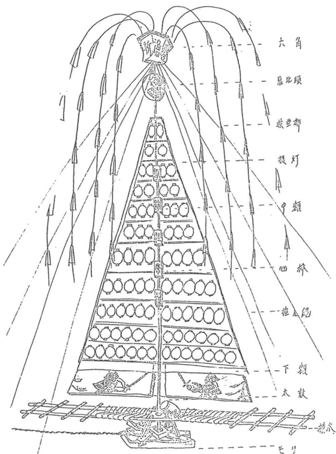
全長(柱) 15.8m 柳(電飾)(6~8本) 8.50m 提網(6~8本)
