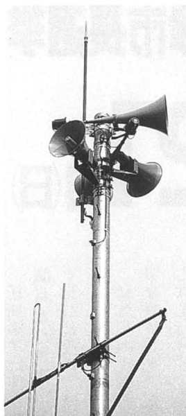
港町公園に設置された防災行政無線。4月から稼働します。
