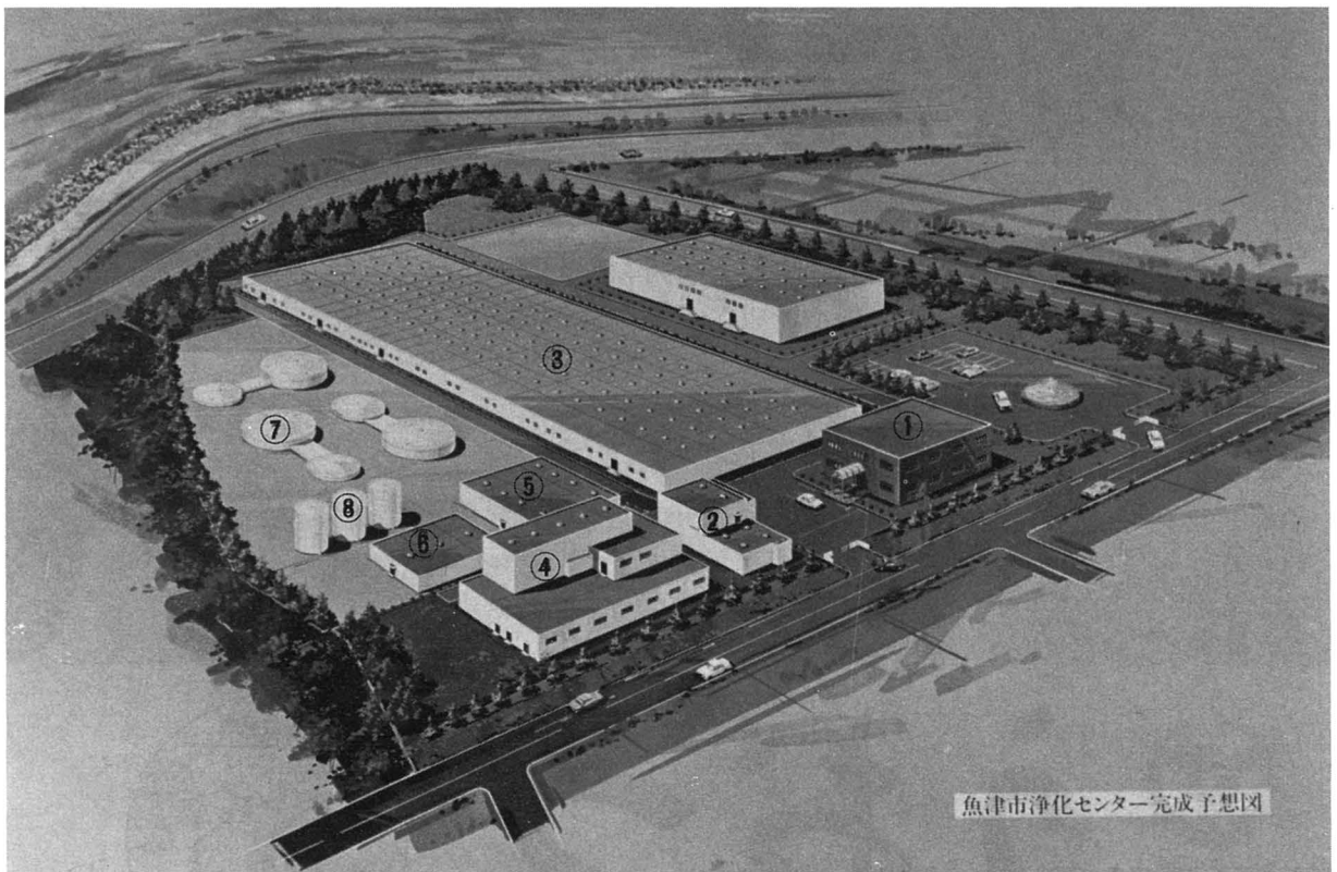
■所在地 魚津市北鬼江地内 ■放流先 富山湾 ①管理棟 ②沈砂池棟 ③水処理棟 ④汚泥処理棟 ⑤汚泥濃縮タンク・ブローア棟 ⑥汚泥洗浄タンク棟 ⑦汚泥消化タンク ⑧ガスホルダー
