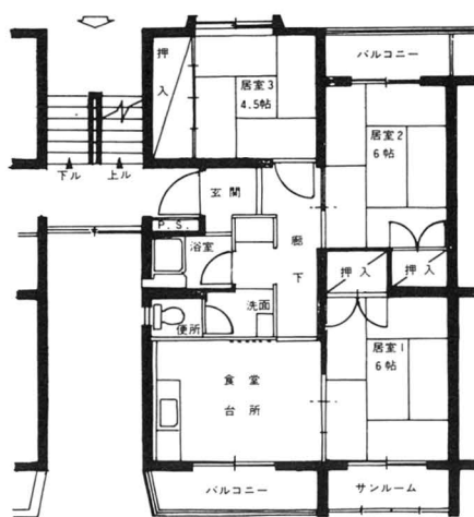
平面図
