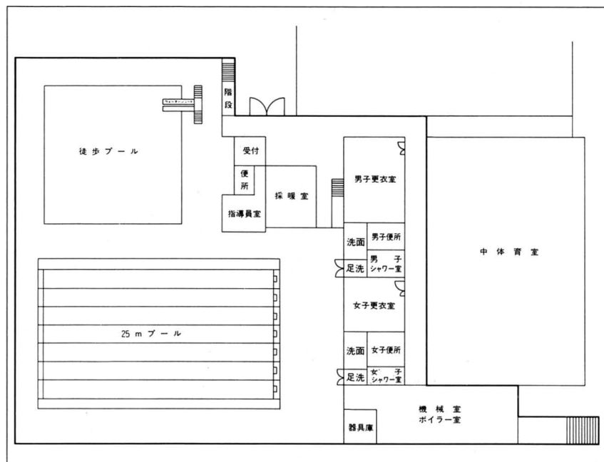
▲温水プール一階平面図
