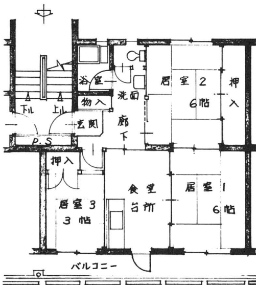
建設する住宅平面図
