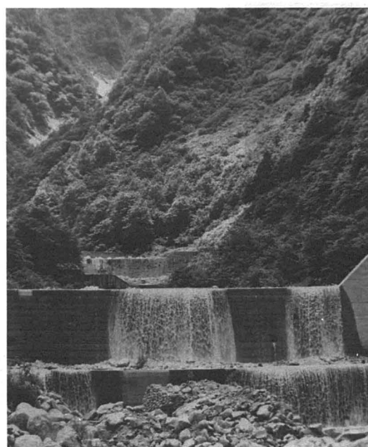
▲東又本流から見た阿部木谷のえん堤
