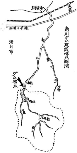
角川治水ダム建設地点略図 角川治水ダム建設地点略図 角川治水ダム建設地点略図
