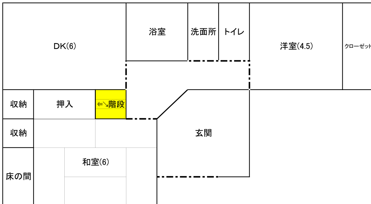
1階間取図
