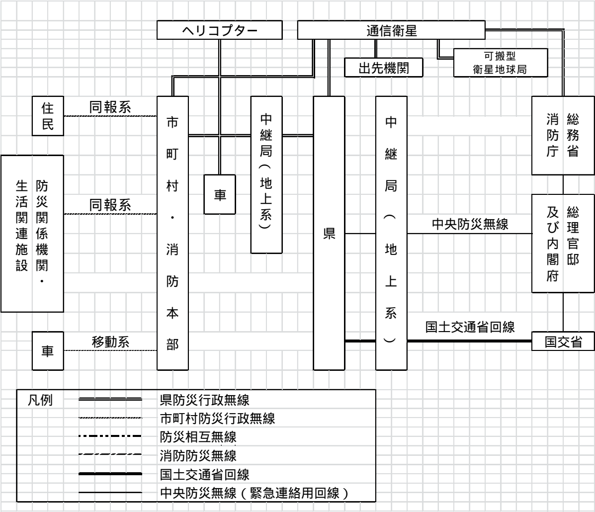
無線通信ネットワーク図
