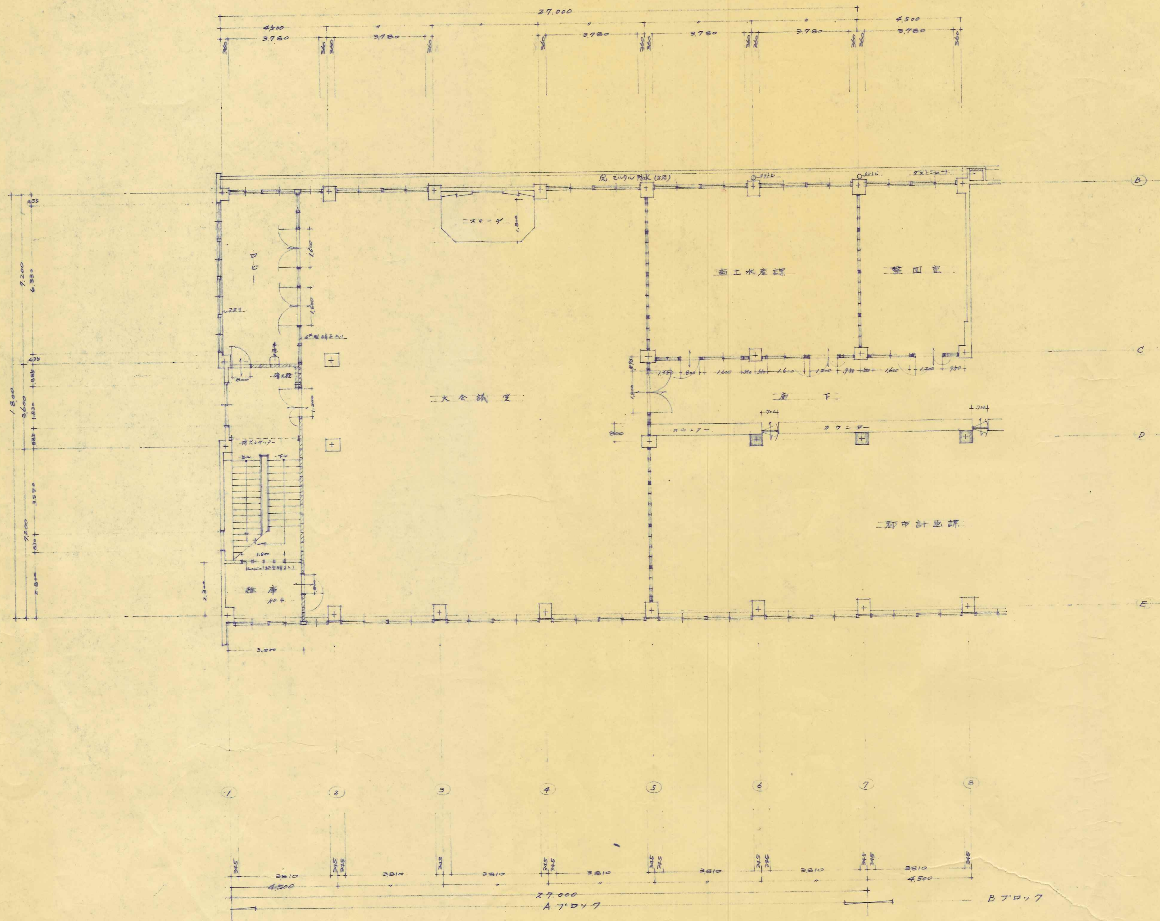
Aブロック 3階平面図 S 1/100
