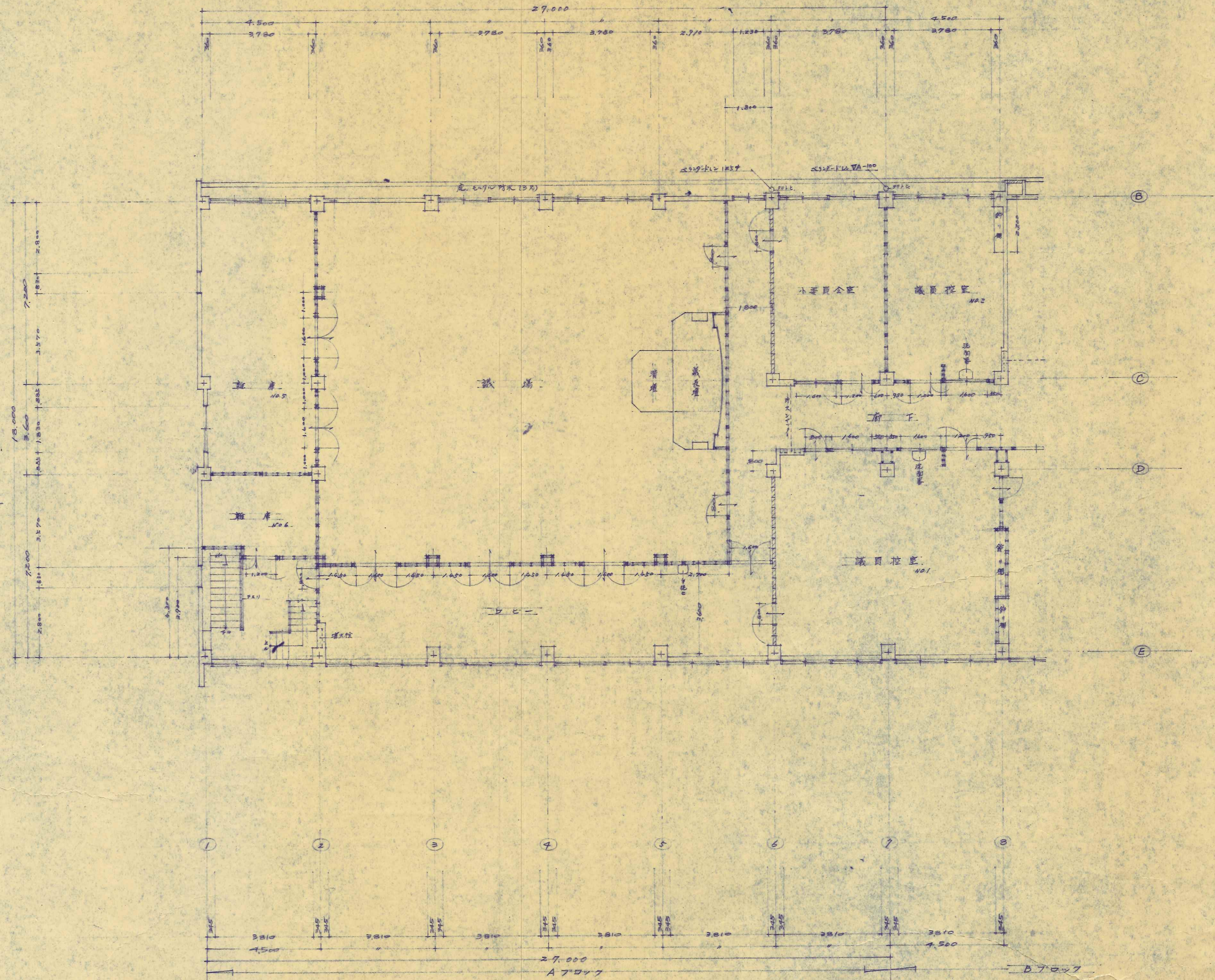
Aブロック 4階平面図 S 1/100
