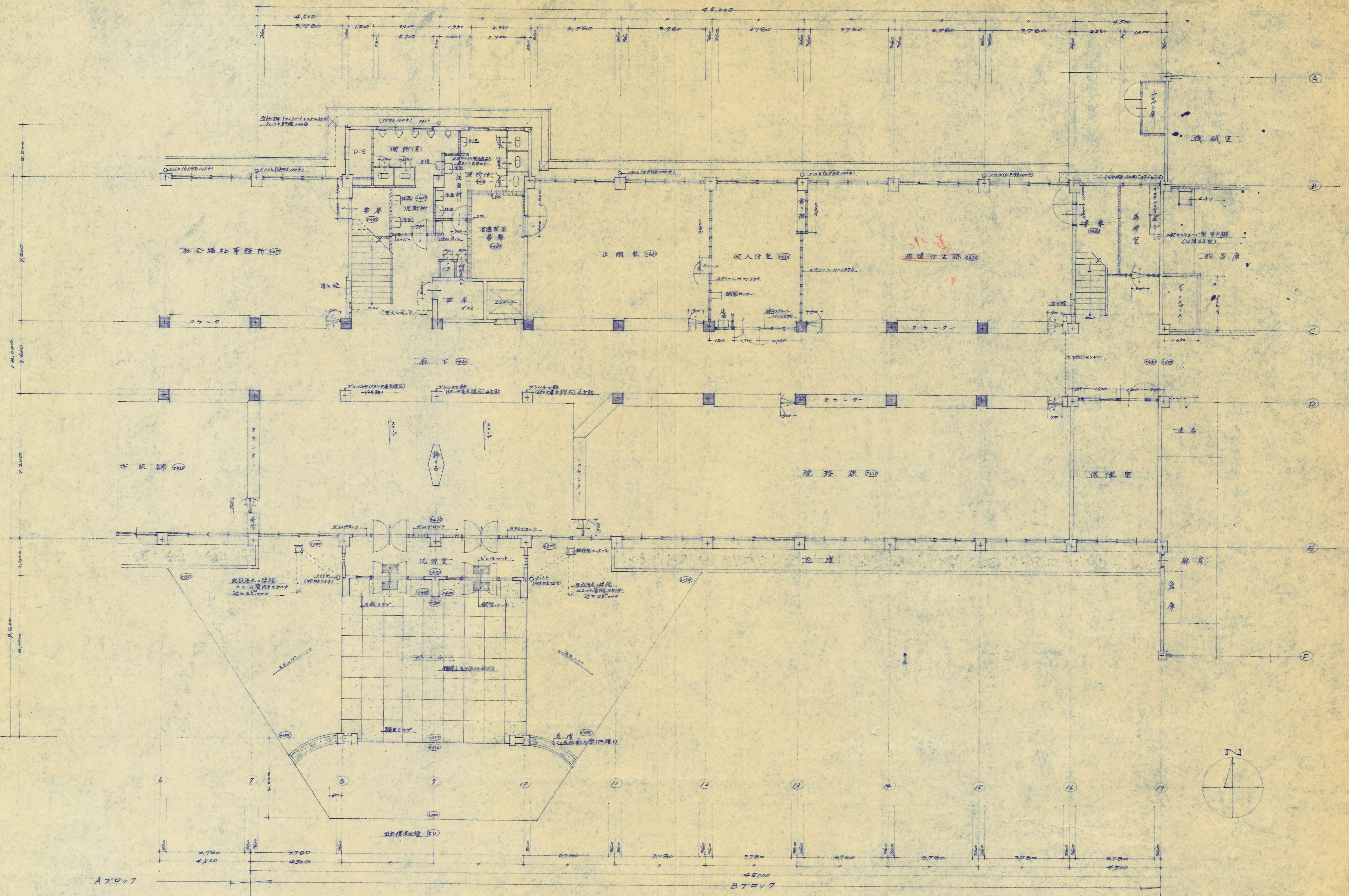
Bブロック 1階平面図 S1/100
