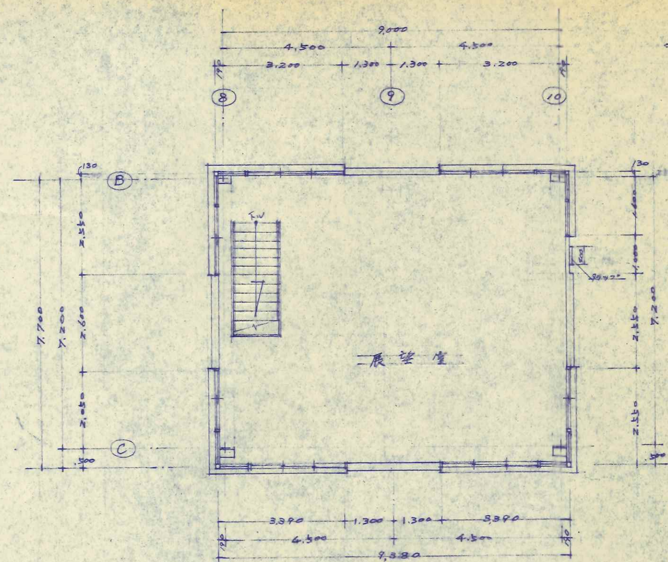
Bブロック塔屋2階平面図 S 1/100
