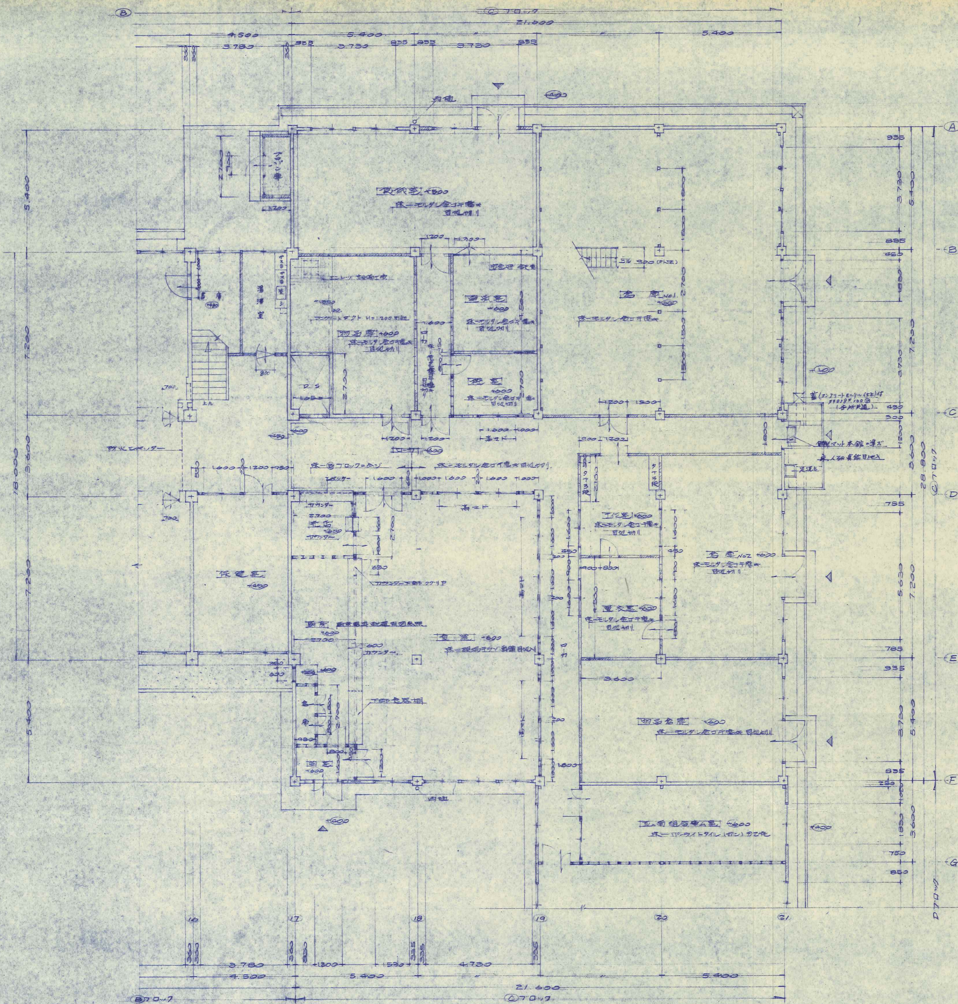
Cブロック1階平面図 S.1/100
