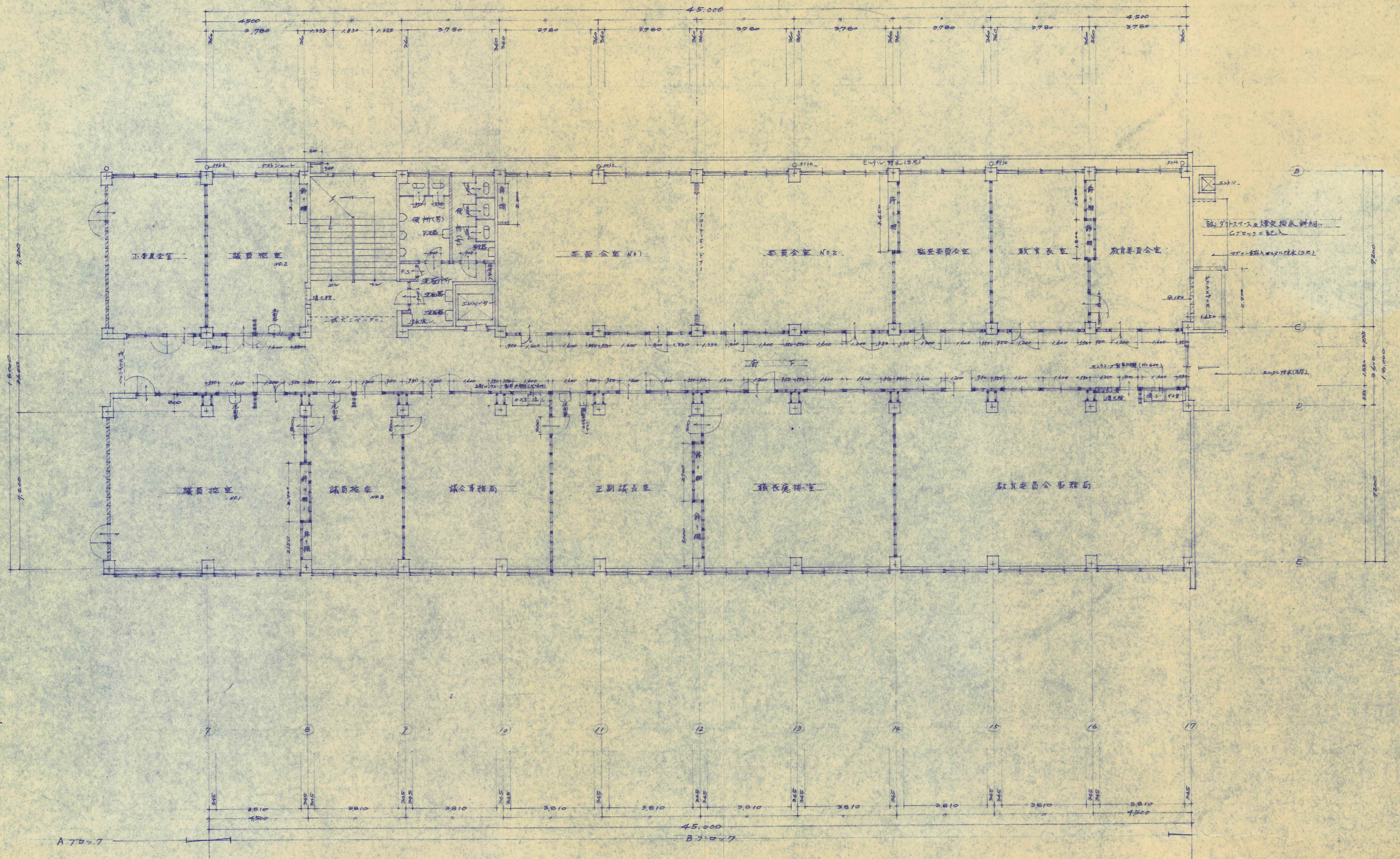
Bブロック 4階平面図 S 1/100
