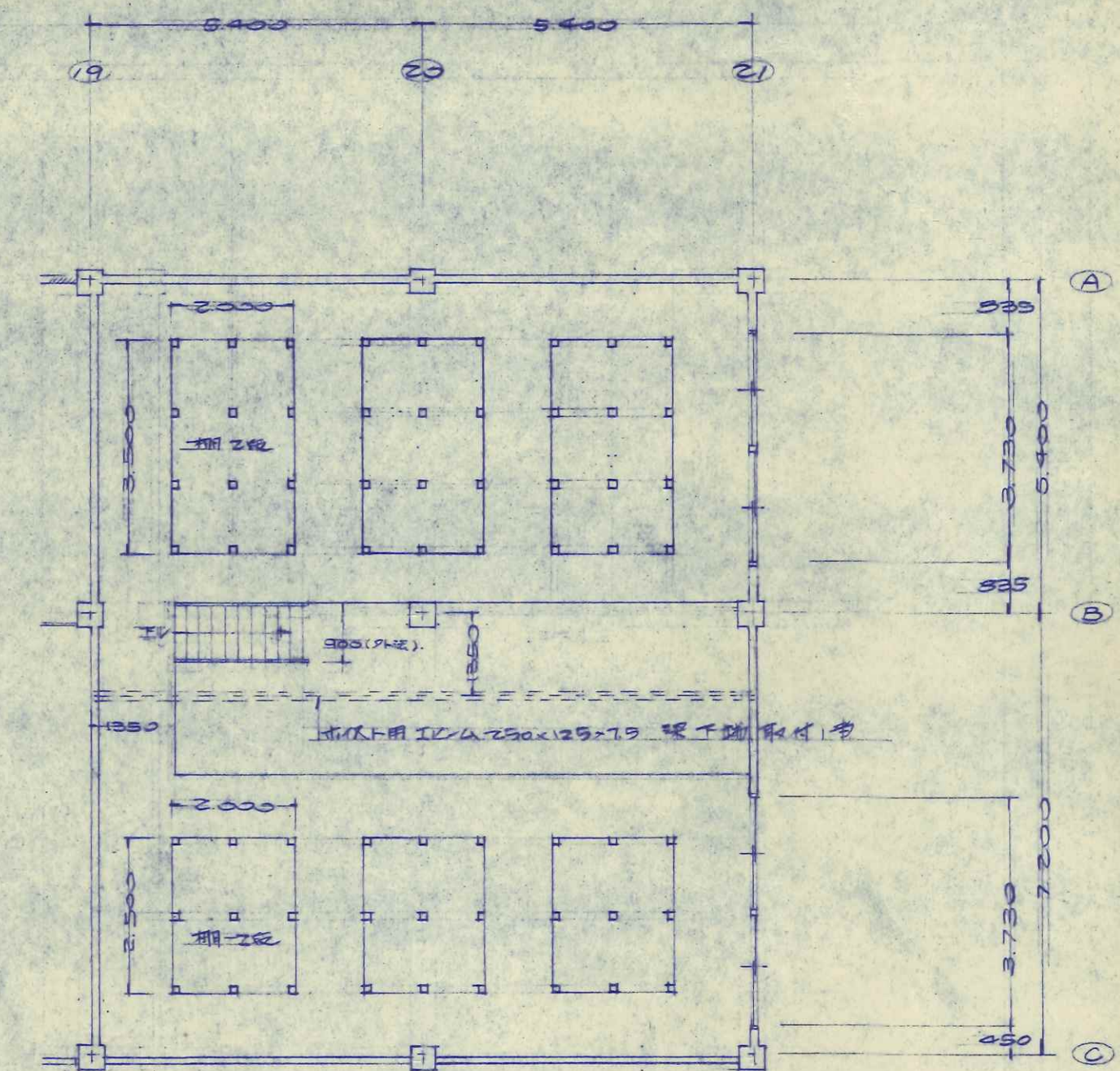
2階平面図 S.2/100
