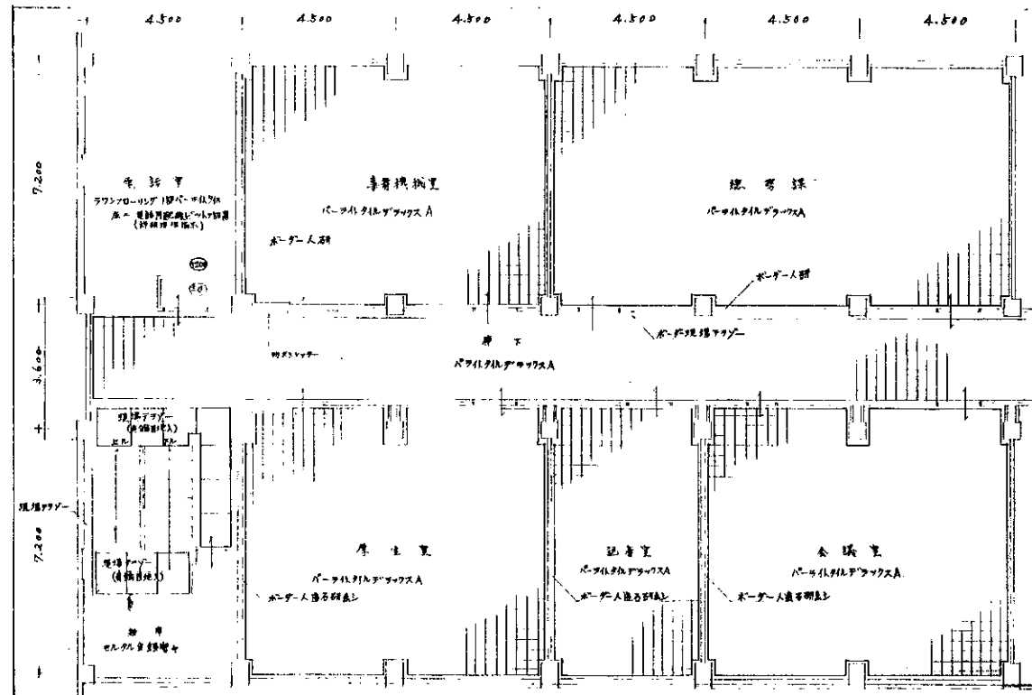
2階床仕上図 1/100
