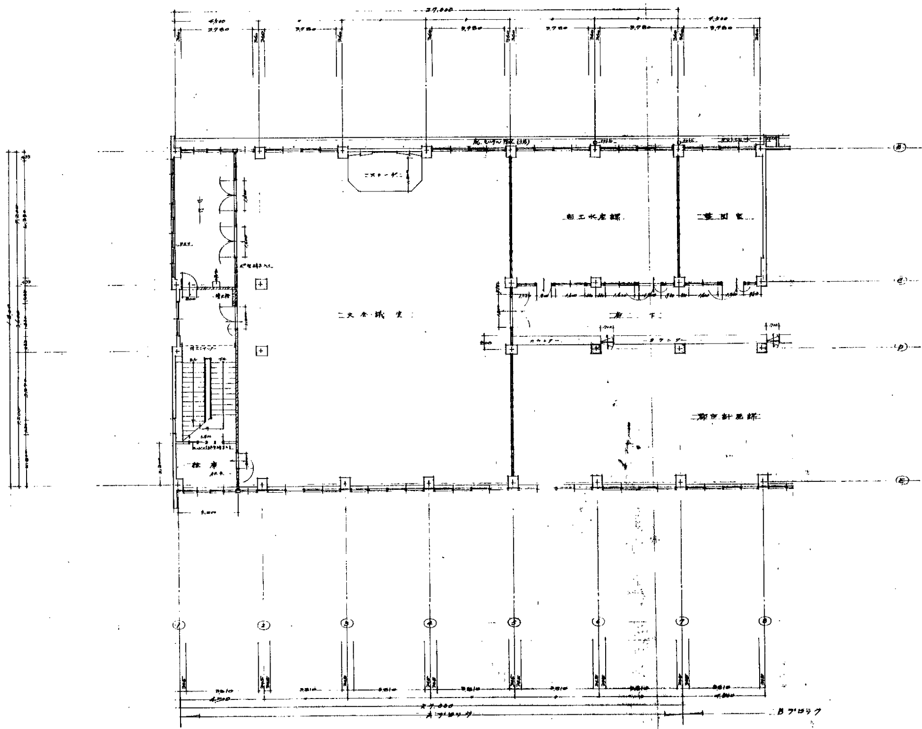
3階平面図 Bブロック
