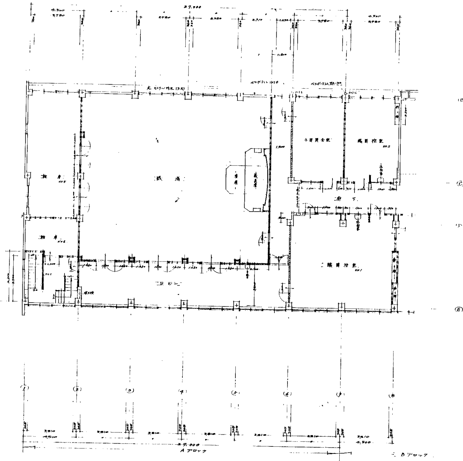
Aブロック 4階平面図 1/100
