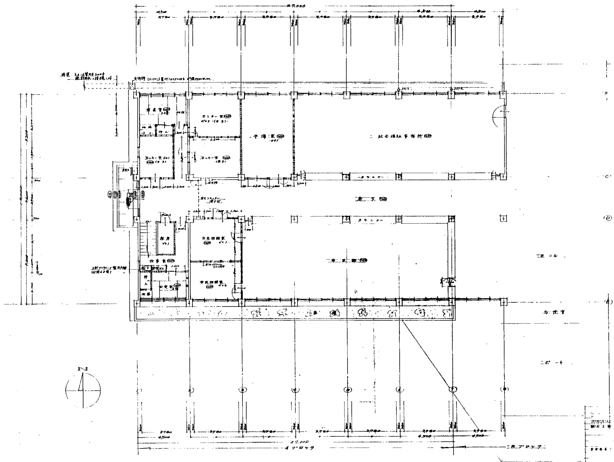
Aブロック 1階平面図 1/100
