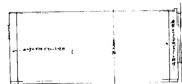
4階断面図 (4階断面図)
