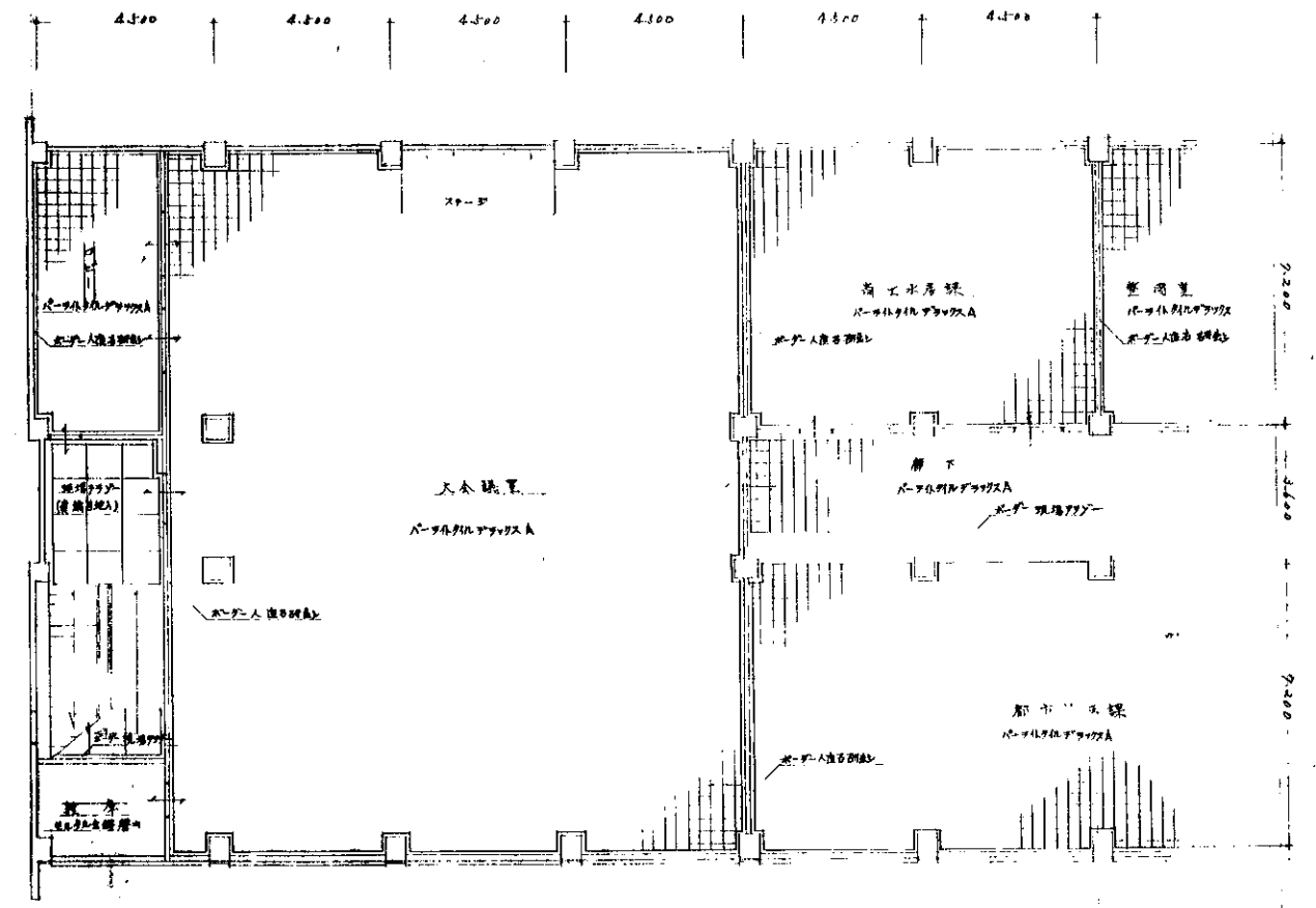
3階床仕上図 S 1/100
