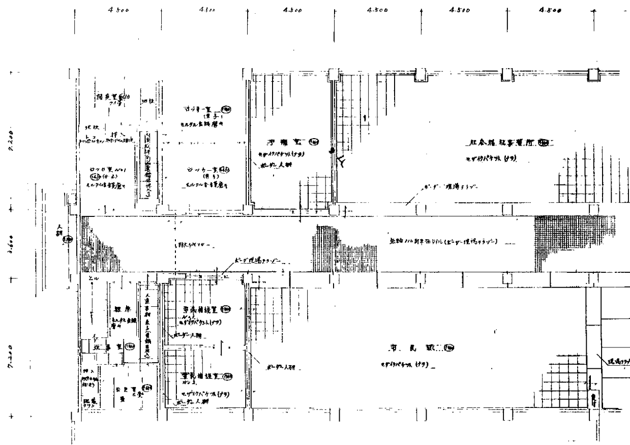
1階床仕上図 S 1/100
