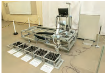
▲開発課題の一例（生産現場の一工程を自動化するモデルシステムの開発）
